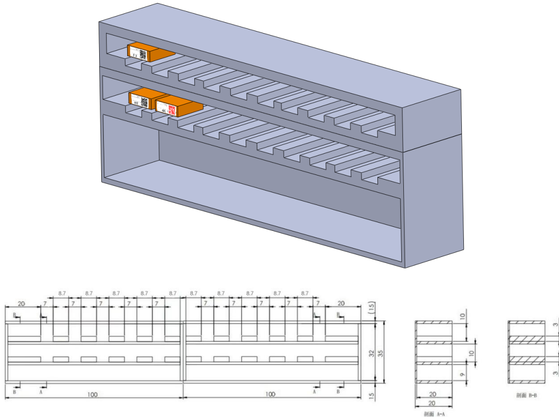
图 5 物流分拣台
